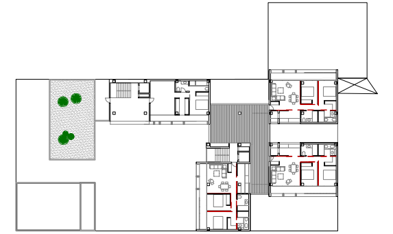
PLANTA CUARTA
